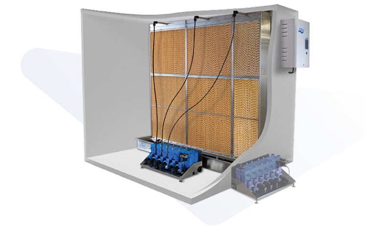
»» Condair ME Humidificación por Evaporación
